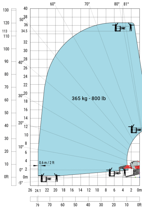
Вращение башни при опущенных аутригерах с платформой 365 кг
